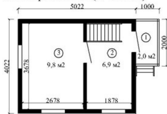
План первого этажа (Н=2430мм)
