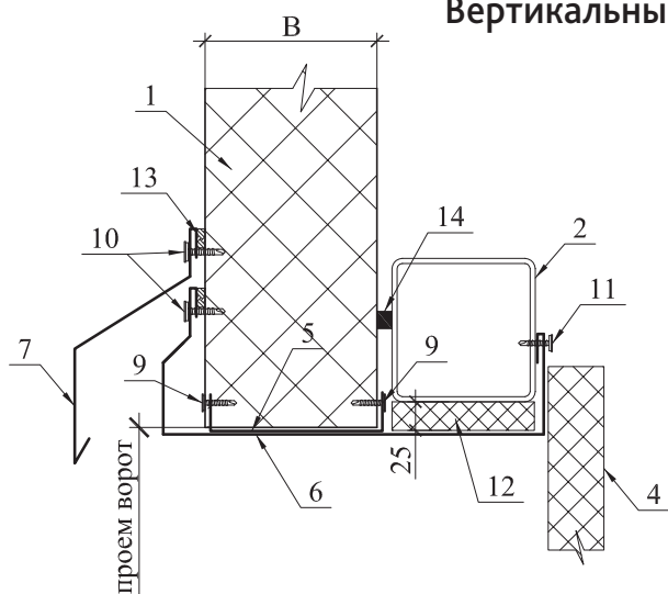
Вертикальный разрез
