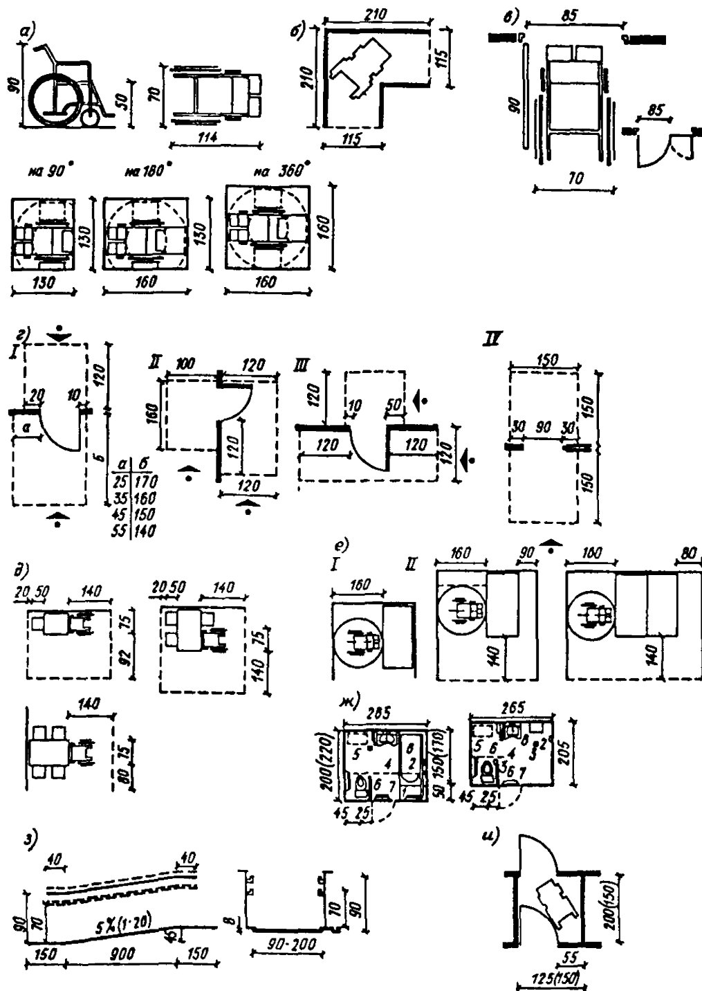
инвалида, не нуждающегося в уходе; II — для инвалида, нуждающегося в уходе; III — для родителей, один из которых инвалид) ж — примеры решения санитарных узлов (I — пересадочная площадка, 2 — настенный смеситель с душевой сеткой на гибком шланге; 3 — трап; 4 — металлический полоз (рельс) на потолке или металлическая штанга для подвески подвижных ручек, лестницы или трапезии, 5 — место для стиральной машины, 6 — опорные поручни, 7 — ручки для закрывания дверей, 8 — откидная скамейка, 3 — размеры пандуса см; и — размеры входного тамбура, см
