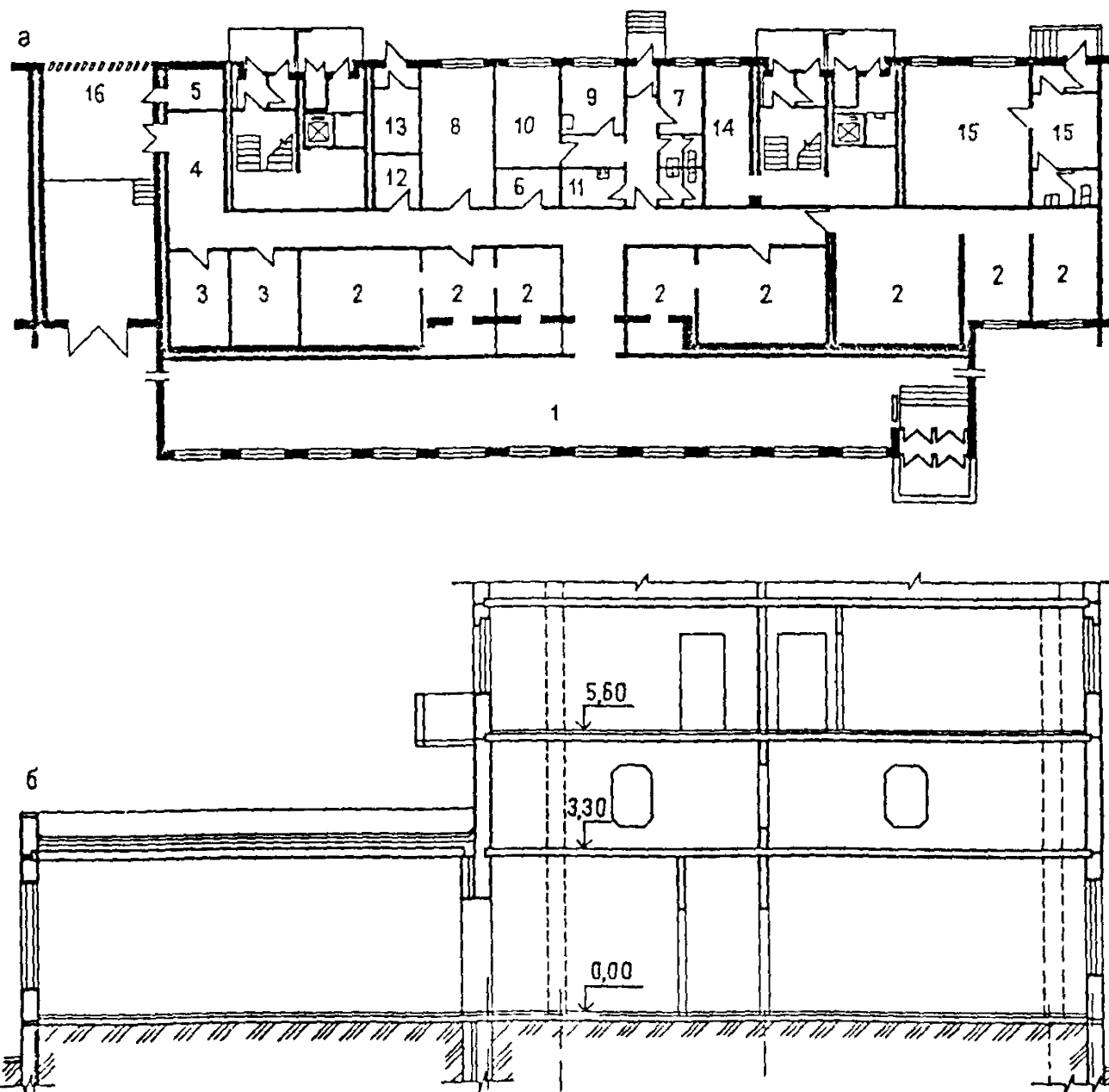
Рис. 25 Встроенно-пристроенный магазин «Книжки» в многоэтажном крупнопанельном жилом доме с выносом объема торгового зала
