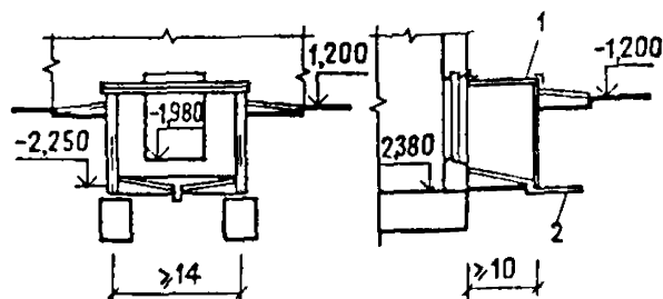
Рис. 27 Устройство приемов перед окнами подвальных и цокольных этажей 1 — съемная решетка, 2 — труба
