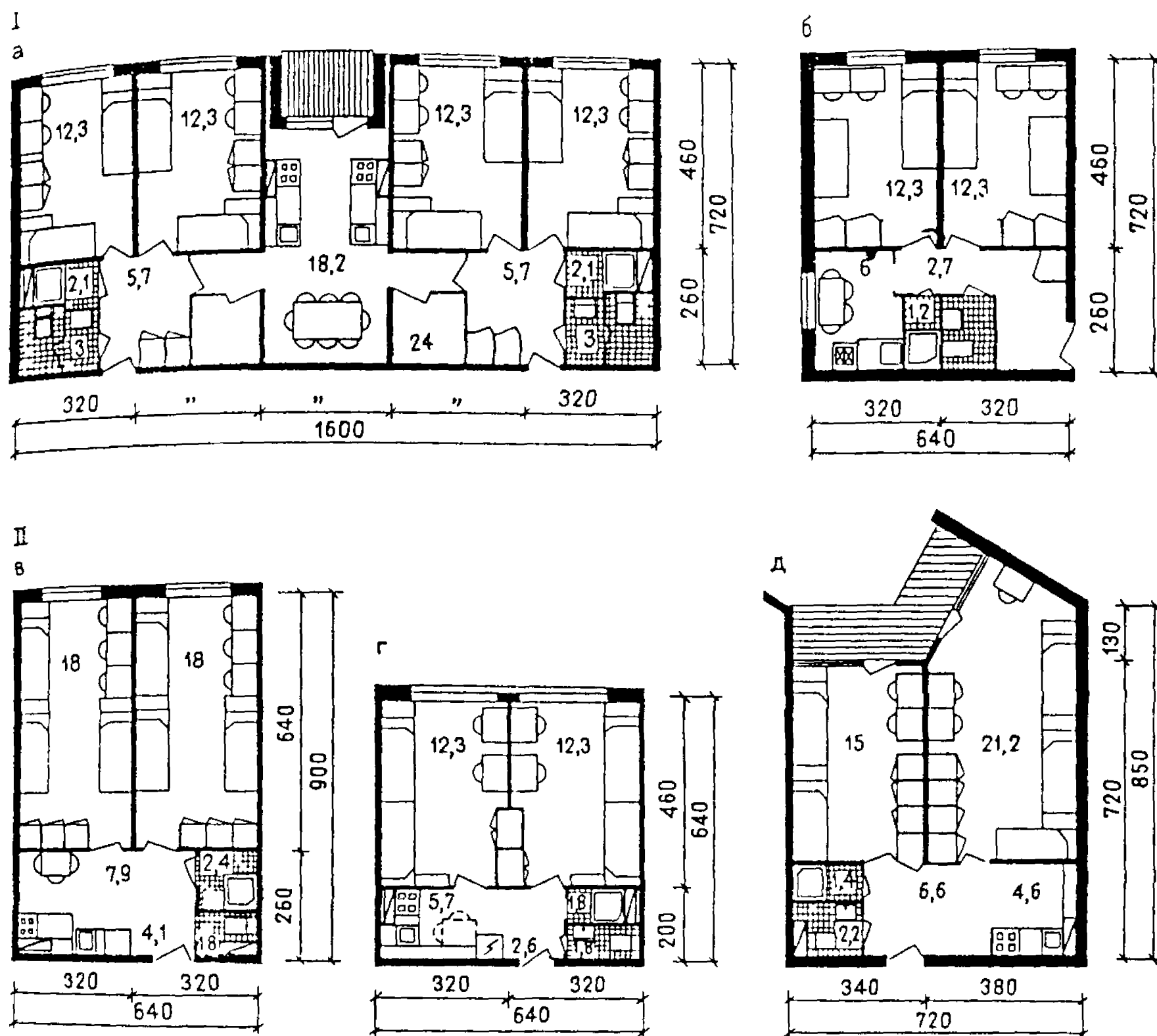
Рис 69 Примеры жилых ячеек общежитий для рабочих и служащих (одиноких) / — жилые ячейки состоящие из жилых комнат передней санитарно гигиенических помещений и кухни с естественным
