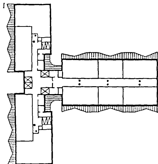
Рис. 15. Здание с галерейной планировочной схемой I — пример планировочной схемы, II — схемы узла вертикальных коммуникаций а — фрагмент плана типового этажа; б — фрагмент плана первого этажа
