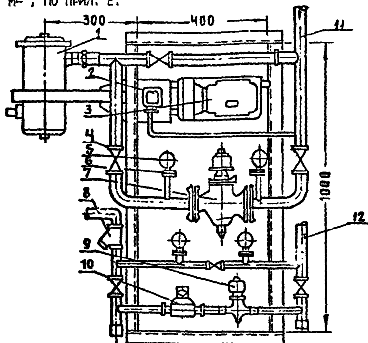
Рис. 5. ПРИМЕР КОМПОНОВКИ ШИТА УПРАВЛЕНИЯ УСТАНОВКИ 'Туман': 1 - компрессор типа МОН; 2 - реле давления РД-1-01; 3 - щиток автоматики; 4 - кран соленоидный муфтовый \varnothing 32 ; 5 - манометр МТ-1; 6 - трехходовой кран КТК; 7 - вентиль СЕМ \varnothing 40 ; 8 - фильтр для воды Ф-1; 9 - вентиль СЕМ \varnothing 15 ; 10 - регулятор давления РДЖ-1А; 11 - трубопровод воздуха к форсункам; 12 - трубопровод воды к форсункам.
