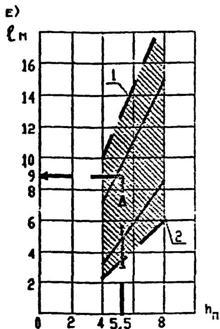
Рис. 3. Максимальный размер помещения или его зоны l = \sqrt{A_n} , м; A_n - площадь помещения или его зоны, обслуживаемая одним воздухоораспределителем, m^2 ; а - компактная струя из плоскостей, рис. 2г, при m = 1,1 ; б - то же, при m = 3,6 ; в - веерная струя, рис. 2е; г - коническая струя, рис. 2д; д - на- стилирующаяся струя из решетки, рис. 2ж, при m = 6 ; 1 - ширина струи 'в' мини- мальная; 2 - ширина струи максимальная; е - настилюющаяся струя из решетки при m = 2,4 ; h_n - высота установки воздухоораспределителя.
