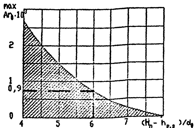
Рис. 4. ПРЕДЕЛЬНОЕ ЗНАЧЕНИЕ КРИТЕРИЯ АРХИМЕДА Ar_0 , ПРИ КОТОРОМ СОХРАНЯЕТСЯ РАСЧЕТНАЯ СХЕМА РАЗВИТИЯ СТРУИ h_n и h_{p,z} - высота помещения и рабочей зоны, d_0 = 1,13 \cdot A_0^{0,5} , ГДЕ A_0 - РАСЧЕТНАЯ ПЛОЩАДЬ ВОЗДУХОРАЗДЕЛИТЕЛЯ, m^2 , ПО ПРИЛ. 2.
