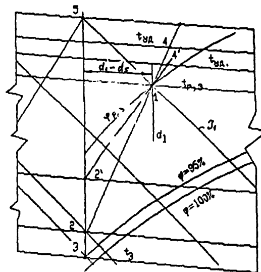
Рис. 1. Схемы процессов приготовления приточного воздуха, построение на T - d диаграмме: а - по адиабатному процессу, б - по политропному процессу, в - по политропному процессу с применением доувлажнения воздуха в помещении.
