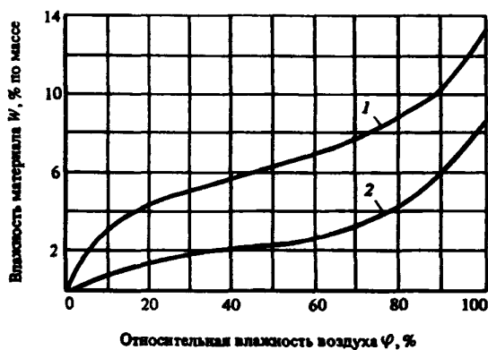
Черт. 9. Зависимость влажности W листового 1 и экструзионного 2 асбестоцемента от относительной влажности воздуха \varphi
