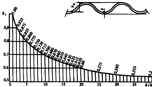
Черт. 7. График для определения коэффициента K_1
