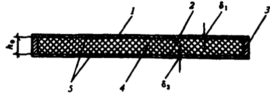
Черт. 5 Поперечное сечение бескаркасной панели с обрамлением
