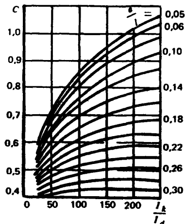
Черт. 6 График для определения коэффициента C
