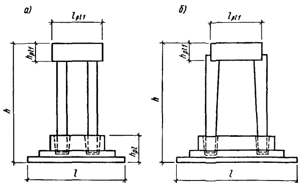
Черт. 4. Сборно-моноплитные фундаменты с подколонниками равного типа
