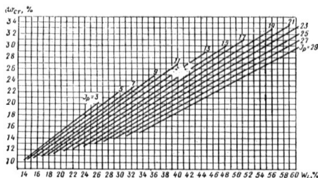
Рис. 5. Значение критической влажности \omega_{cr} в зависимости от числа пластичности I_P и границы текучести \omega_L грунта
