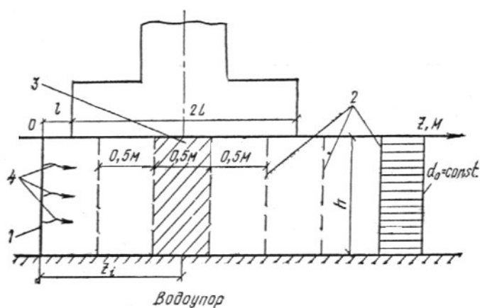
Рис. 73. Схема для расчета расселения основания при горизонтальной фильтрации
