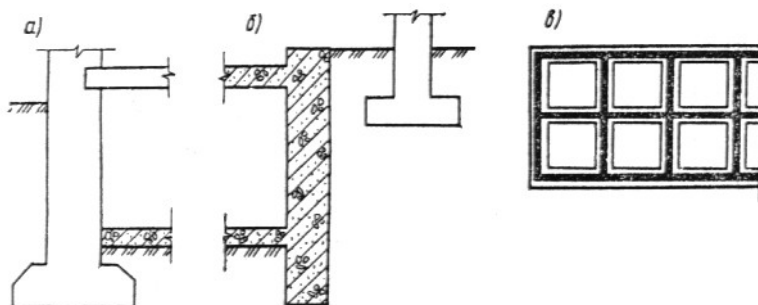
Рис. 26. Конструктивные мероприятия, препятствующие смещению фундаментов
