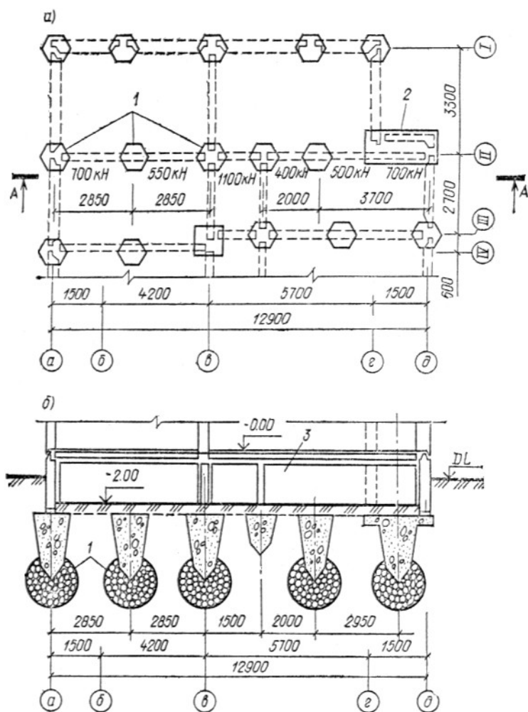
Рис. 55. Столбчатые фундаменты вытрамбованных котлованах с уширением основания
