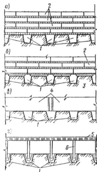
Рис. 53. Конструкция ленточных прерывистых фундаментов
