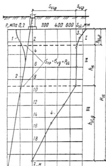
Рис. 35. Зоны деформации просадочного грунта в основании фундамента
