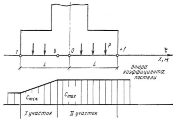
Рис. 74. Схема расчета деформаций при горизонтальной фильтрации
