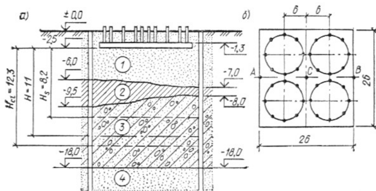
Рис. 21. Геологический разрез (а) и план фундаментной плиты (б) к примеру расчета деформаций основания
