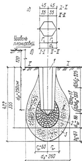
Рис. 56. Фундамент с уширением основания
