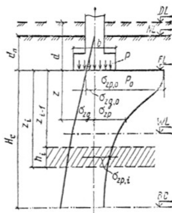
Рис. 14. (1 прил. 2). Схема распределения вертикальных напряжений в линейно-деформируемом полупространстве.
