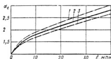
Рис. 24. Пример зависимости предельных значений степени изменчивости сжимаемости основания \alpha_E от среднего значения модуля деформации грунтов основания в пределах плана здания
