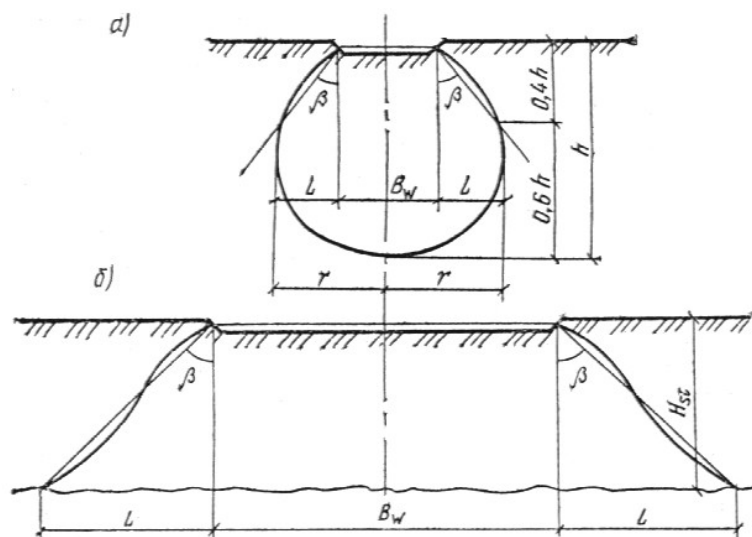
Рис. 37. Схемы увлажненных зон при замачивания грунтов
