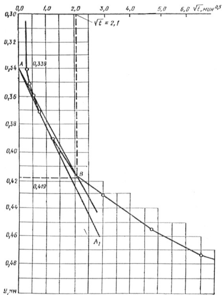
Рис. 66. График для определения коэффициента консолидации
