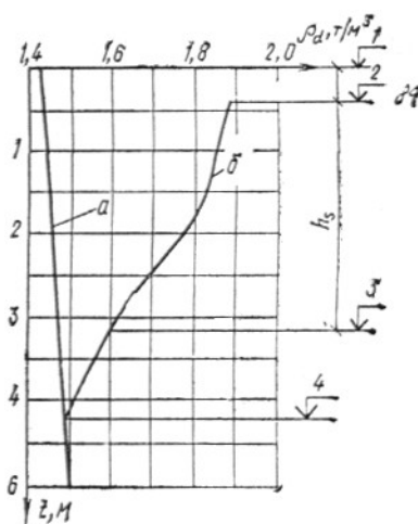
Рис. 50. Изменение плотности грунтов по глубине до уплотнения (а) и после уплотнения тяжелыми трамбовками (б)
