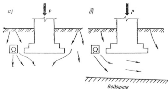
Рис. 69. Схемы замачивания основания фундаментов
