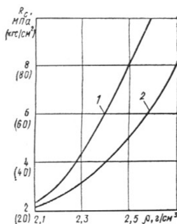
Рис. 67. Зависимость прочности выветрелых скальных грунтов, образованных из кварце содержащих (1) и бескварцевых (2) пород, от их плотности
