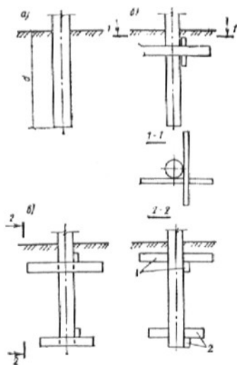
Рис. 81. Схема закреплений стоек в грунте с различной установкой ригелей:
