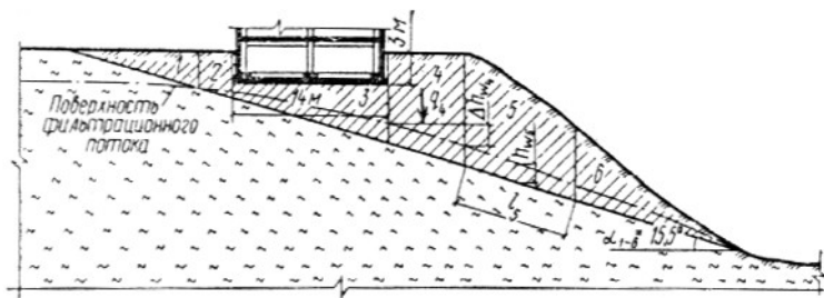
Рис. 32. Схема к примеру расчета несущей способности основания при возможном сдвиге по плоской поверхности
