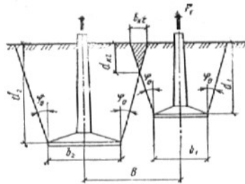
Рис. 79. Схема к расчету устойчивости при выдергивании близко расположенных фундаментов
