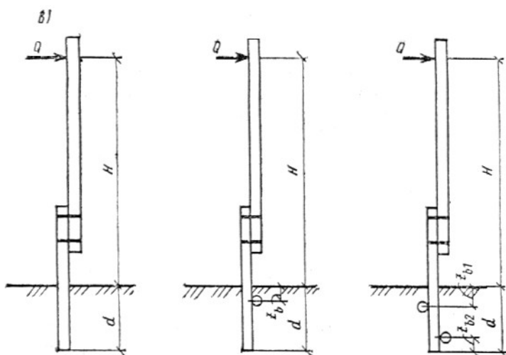
Рис. 85. Схемы к расчету стоек деревянных опор в грунте а - схема выдергивания; б - схема определения расчетной ширины элемента стойки; в - расчетная схема закрепления
