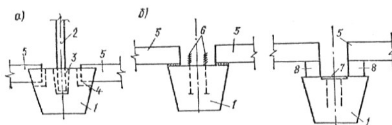
Рис. 52. Сопряжение колонн с фундаментом в вытрамбованном котловане
