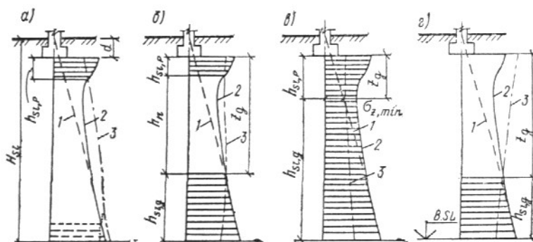
Рис. 42 (4 прил. 2). Схемы к расчету просадок основания
