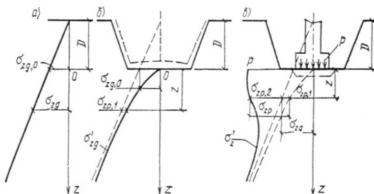
Рис. 18. Эпюры давлений
