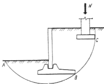
Рис. 29. Схема потери устойчивости основания системы «подпорная стенка - фундамент»
