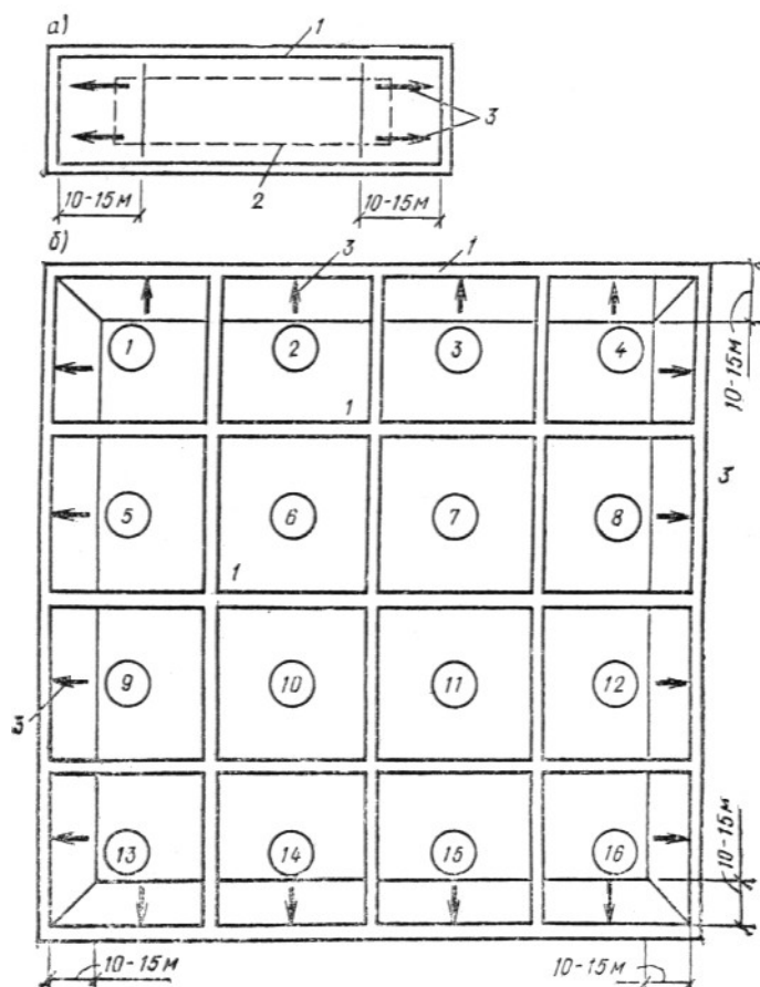
Рис. 58. Схема планировки котлованов и карт для замачивания
