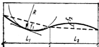
Рис. 8. Схема прогиба (выгиба) сооружения: \frac{f_1}{L_1} - относительный прогиб на участке L_1 ; \frac{f_2}{L_2} - относительный выгиб на участке L_2 ; \rho наибольшая кривизна
