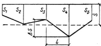
Рис. 6. Схема осадок основания сооружения. \frac{\Delta s}{L} - относительная неравномерность осадок соседних фундаментов
