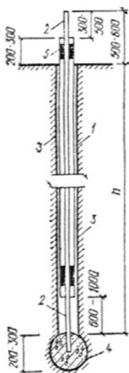
Рис. 41. Конструкция глубинной марки
