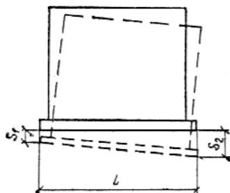
Рис. 7. Схема крена жесткого сооружения i = \frac{s_2 - s_1}{L}
