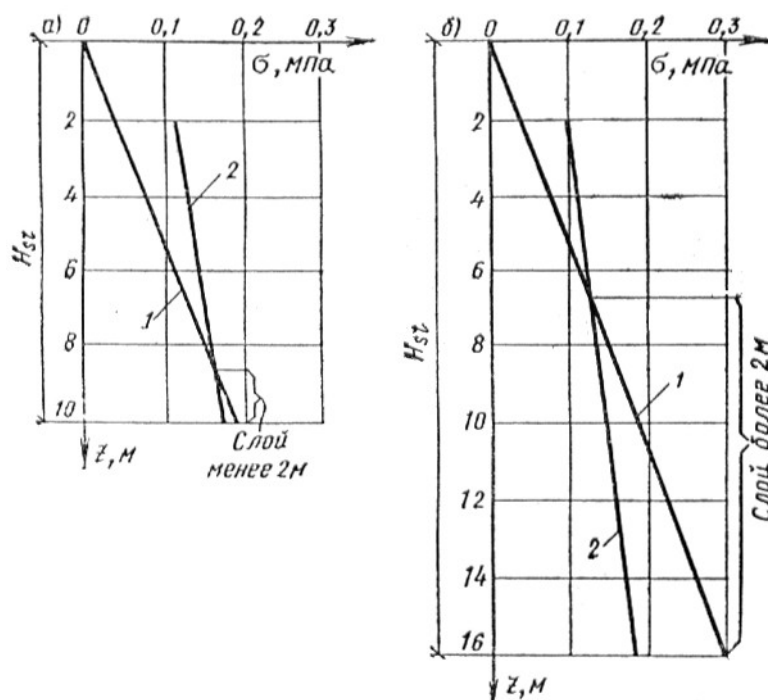
Рис. 38. Пример определения типа грунтовых условий по изменению напряжения от собственного веса грунта \sigma_{z,g} (1) и начального просадочного давления P_{sl} (2) по глубине просадочной толщи;
