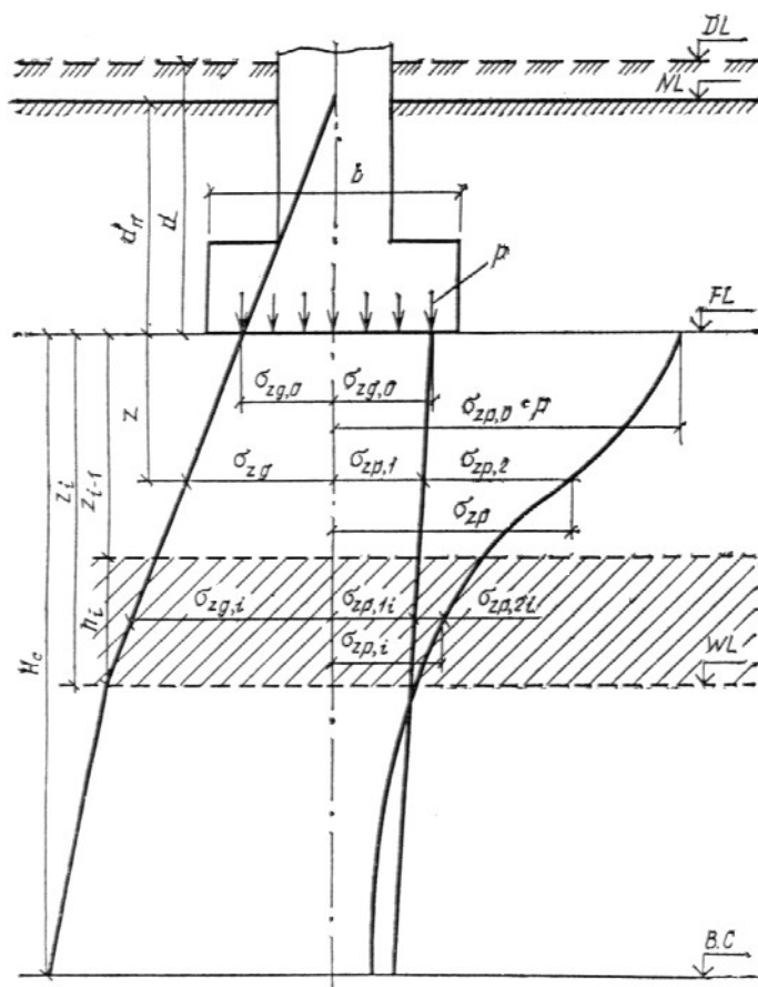
Рис. 19. Схема расчета осадки фундамент
