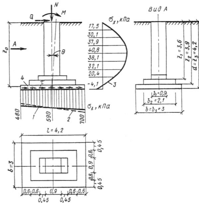
Рис. 23. Схема к примеру расчета крена заглубленного фундамента
