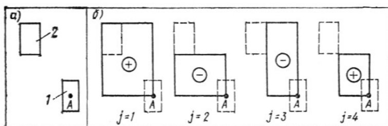
Рис 15. (2 прил. 2). Схема к определению дополнительных вертикальных напряжений \sigma_{zp,\alpha} в основании рассчитываемого фундамента с учетом влияния соседнего фундамента методом угловых точек
