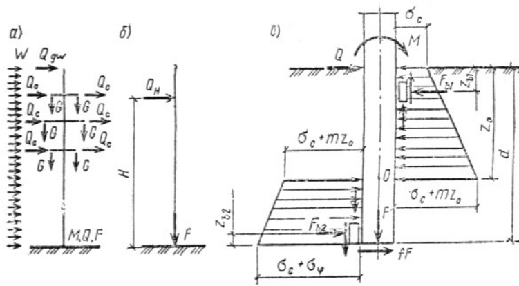
Рис. 83. Схема к расчету стоек на опрокидывание
