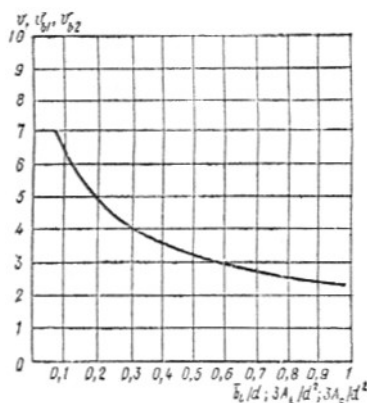
Рис. 84. График зависимости коэффициентов v = f\left(\frac{b_l}{d}\right)
