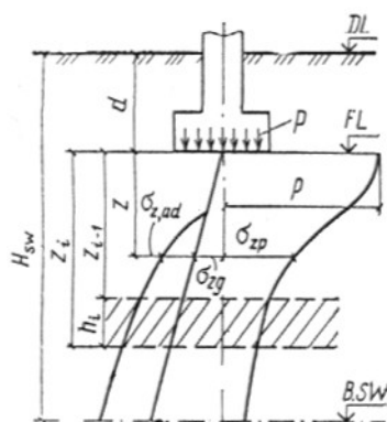
Рис. 62. Схема к расчету подъема основания при набухании грунта
