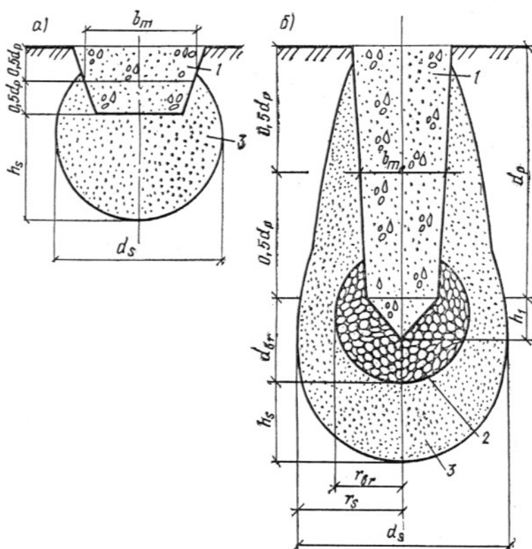
Рис. 51. Фундаменты в вытрамбованных котлованах
