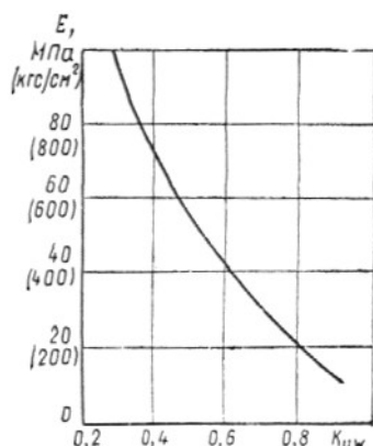
Рис. 68. Зависимость модуля деформации от степени выветрелости грунта
