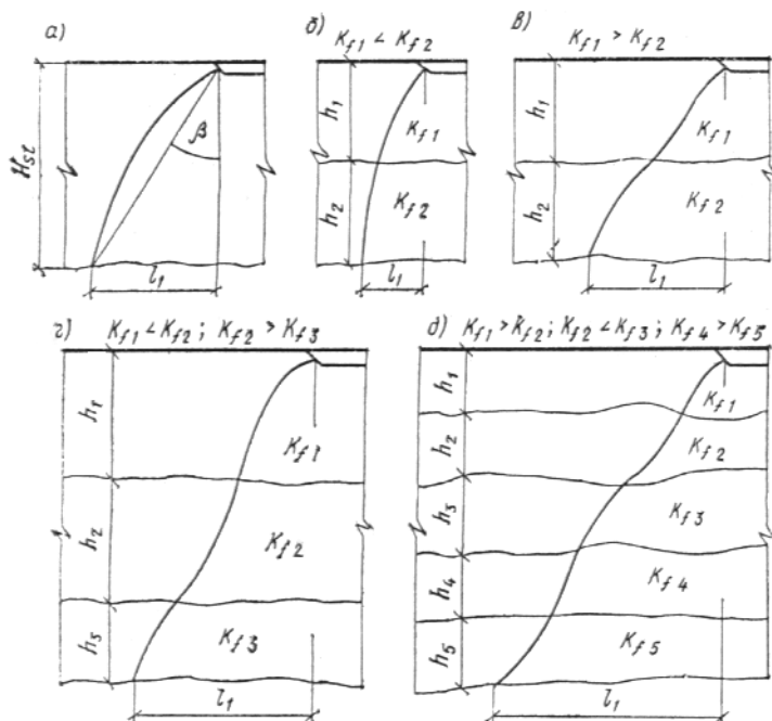
Рис. 45. Схемы распространения увлажнения в стороны от источника замачивания в толщах лессовых грунтов при различном их напластовании
