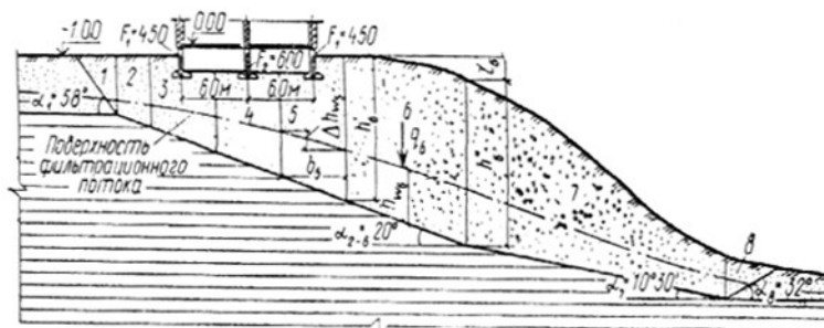
Рис. 33. Схема к примеру расчета несущей способности основания при возможном сдвиге по ломаной поверхности
