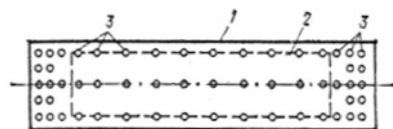
Рис. 59. Рекомендуемая схема расположения скважин для замачивания котлованов
