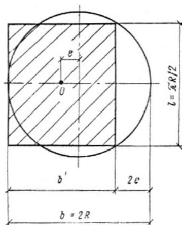
Рис. 28. Схема для определения приведенных размеров круглого фундамента
