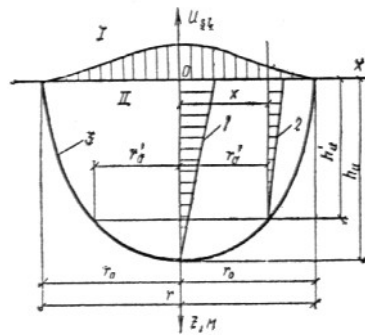
Рис. 48. Расчетная схема для определения горизонтальных перемещений в массиве грунта
