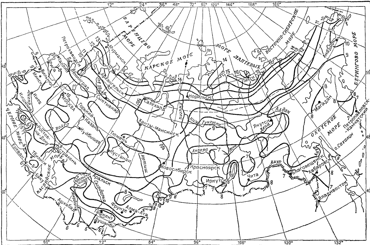
Рис. Схематическая карта изолиний постоянной величины T для определения температуры воздуха на- более жарких суток
