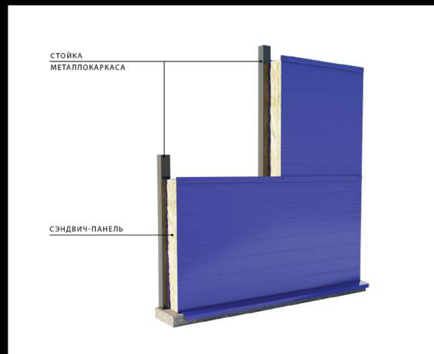
МОНТАЖ СЭНДВИЧ-ПАНЕЛЕЙ
