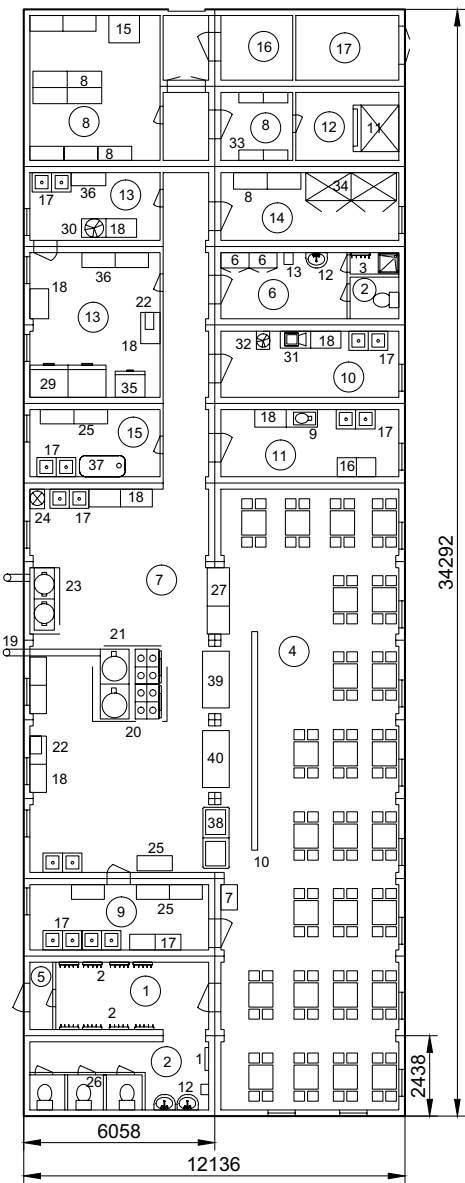
Столовая на 100 посадочных мест
