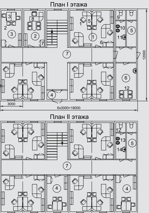
Офисное здание на 35 рабочих мест
